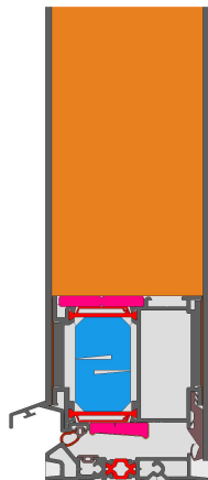
Berechnungsmodell
