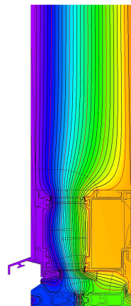
Isothermengrafik
